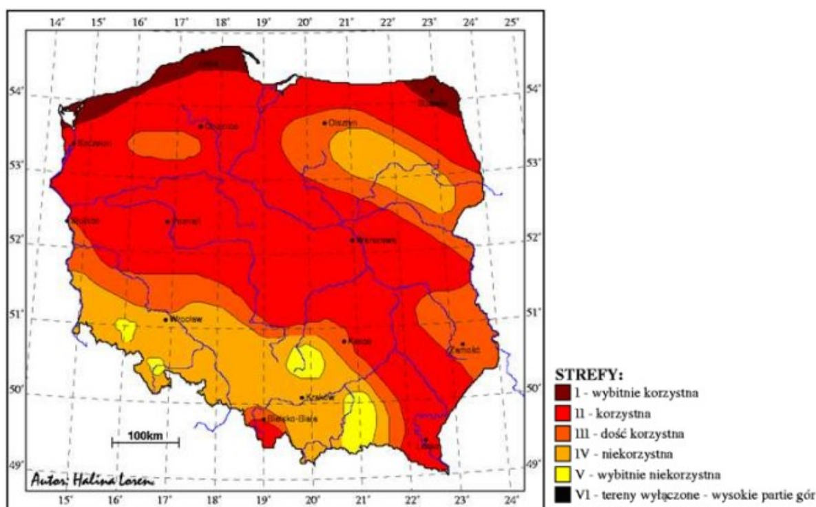
RYСУNEK 6. STREFY ENERGETYCZNE W POLSCE.
